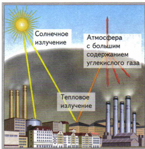
Рис. 51. Парниковый эффект
